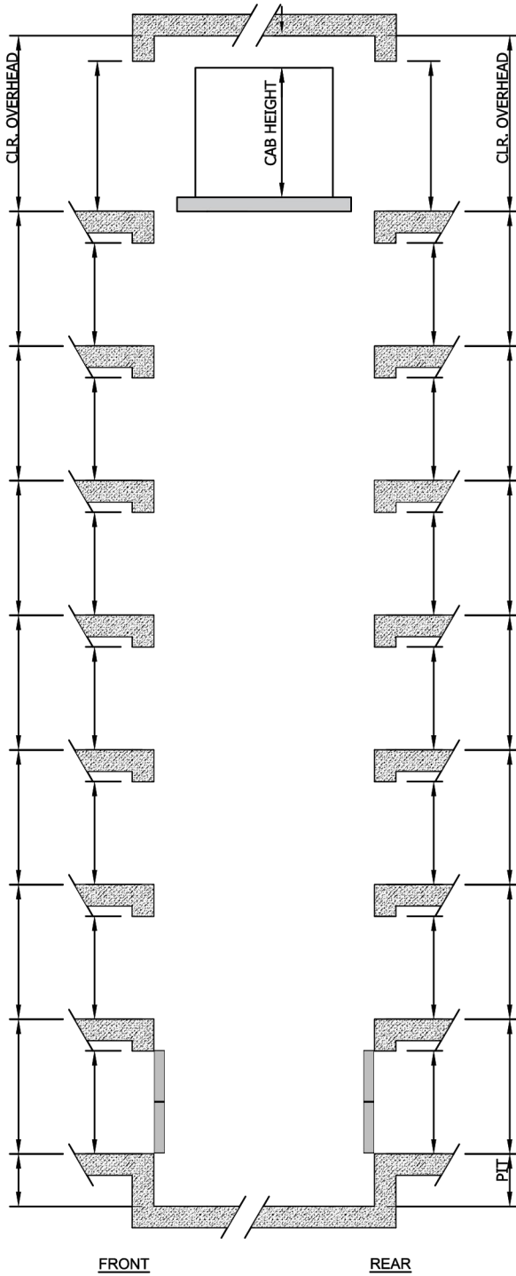
ELEVATION
