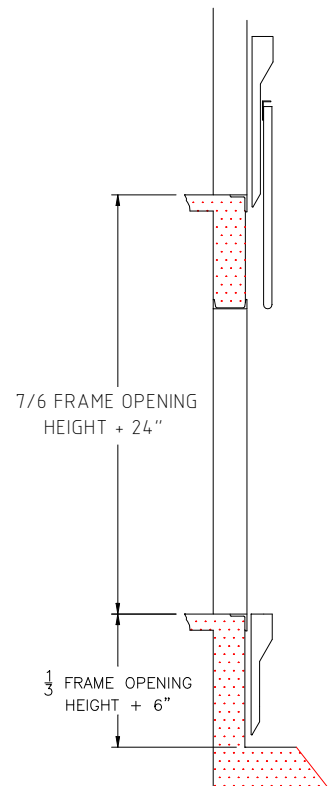
ELEVATION
