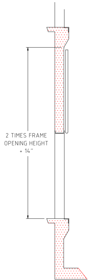
ELEVATION
