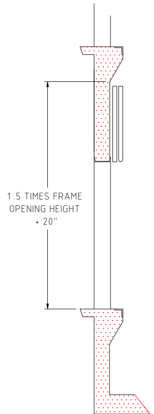
ELEVATION
